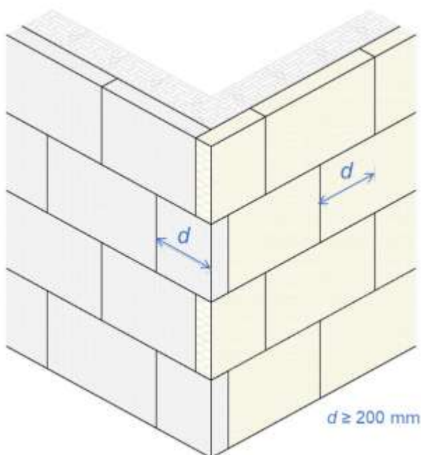
Figure 3. Juxtaposition avec le système Baunit ProSystem / PSE : jonction en angle sortant entre les panneaux en PSE et les panneaux en laine de roche
