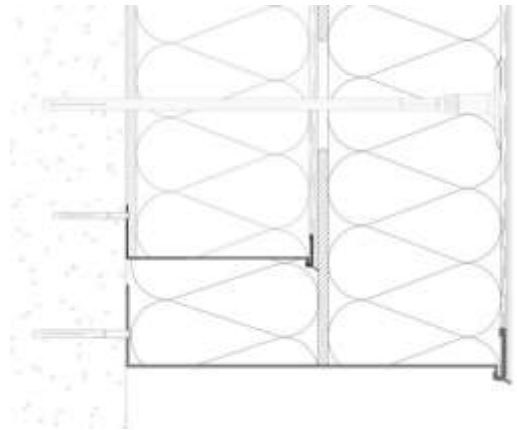
4b : nouveau profilé de départ sans dépose de l'existant
