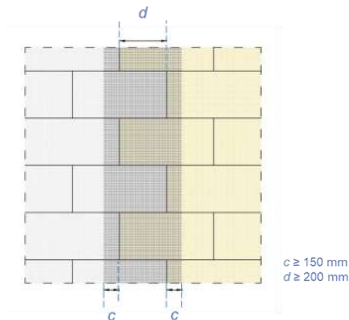
Figure 2a. Juxtaposition avec le système Baunit ProSystem / PSE : jonction en façade entre les panneaux en PSE et les panneaux en laine de roche.
