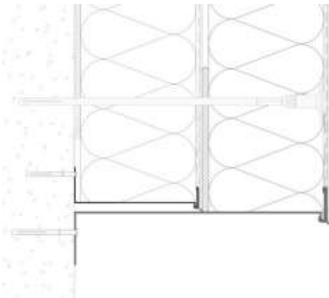
4c : nouveau profilé de départ inversé sans dépose de l'existant
