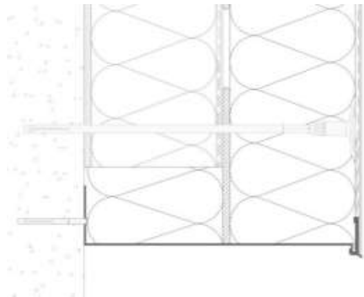
4d : nouveau profilé de départ après élimination de l'existant
