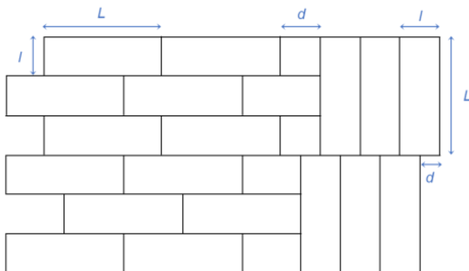
Figure 1a. Principe de juxtaposition des poses horizontale et verticale des panneaux isolants de dimensions 1200 × 600 mm.
