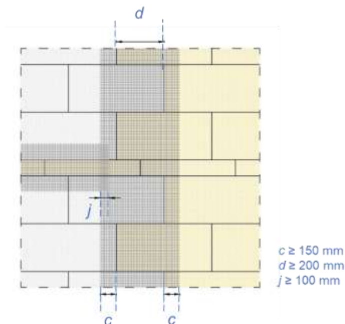
Figure 2b. Juxtaposition avec le système Baunit ProSystem / PSE : jonction en façade entre les panneaux en PSE et les panneaux en laine de roche, avec bande filante.
