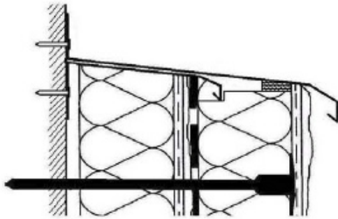
Figure 2a : nouvelle couverte inversée sans dépose de l'existant
